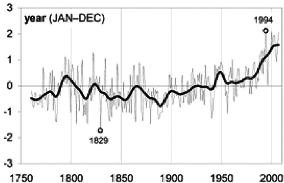
Figure 1. Evolution moyenne des températures dans les Alpes
