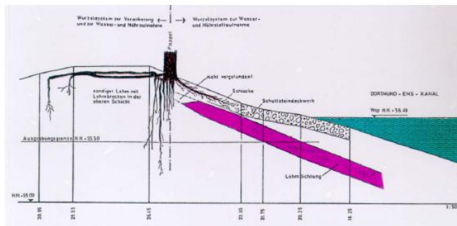
Querschnitt
